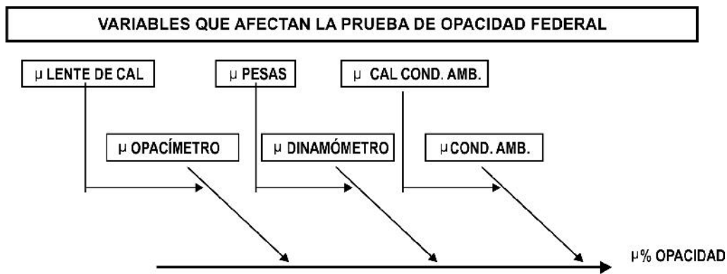
Figura 1. Prueba de Ciclo de Opacidad Federal
